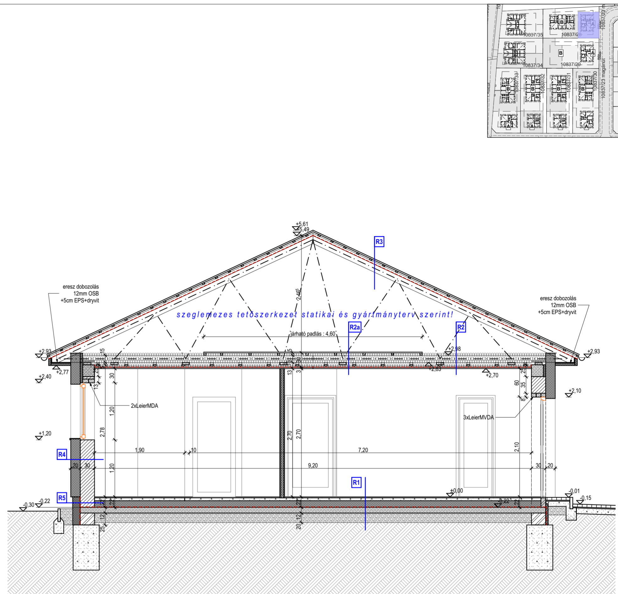
M29A-1 Metszet 1:50
