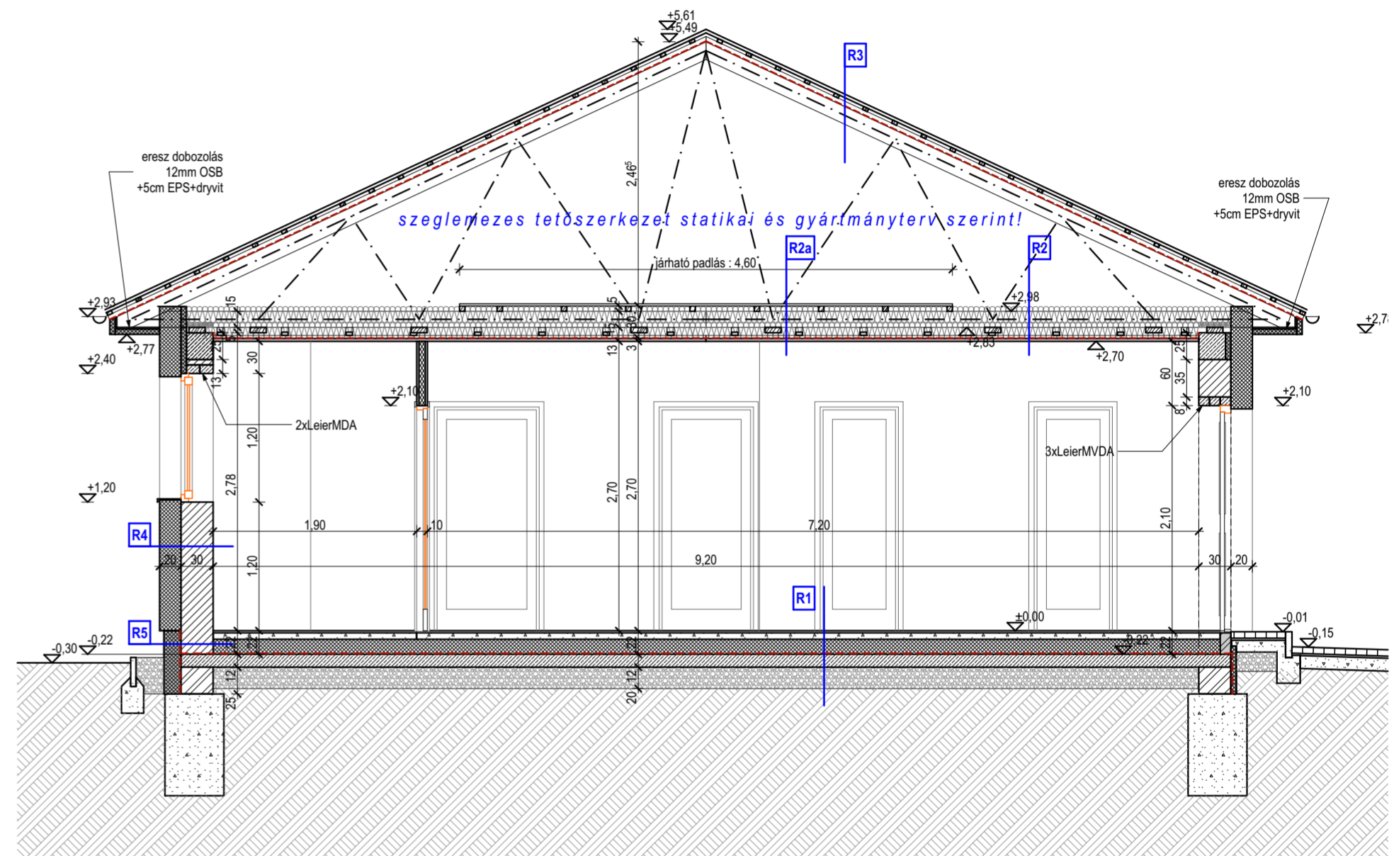
M28A-1 Metszet 1:50
