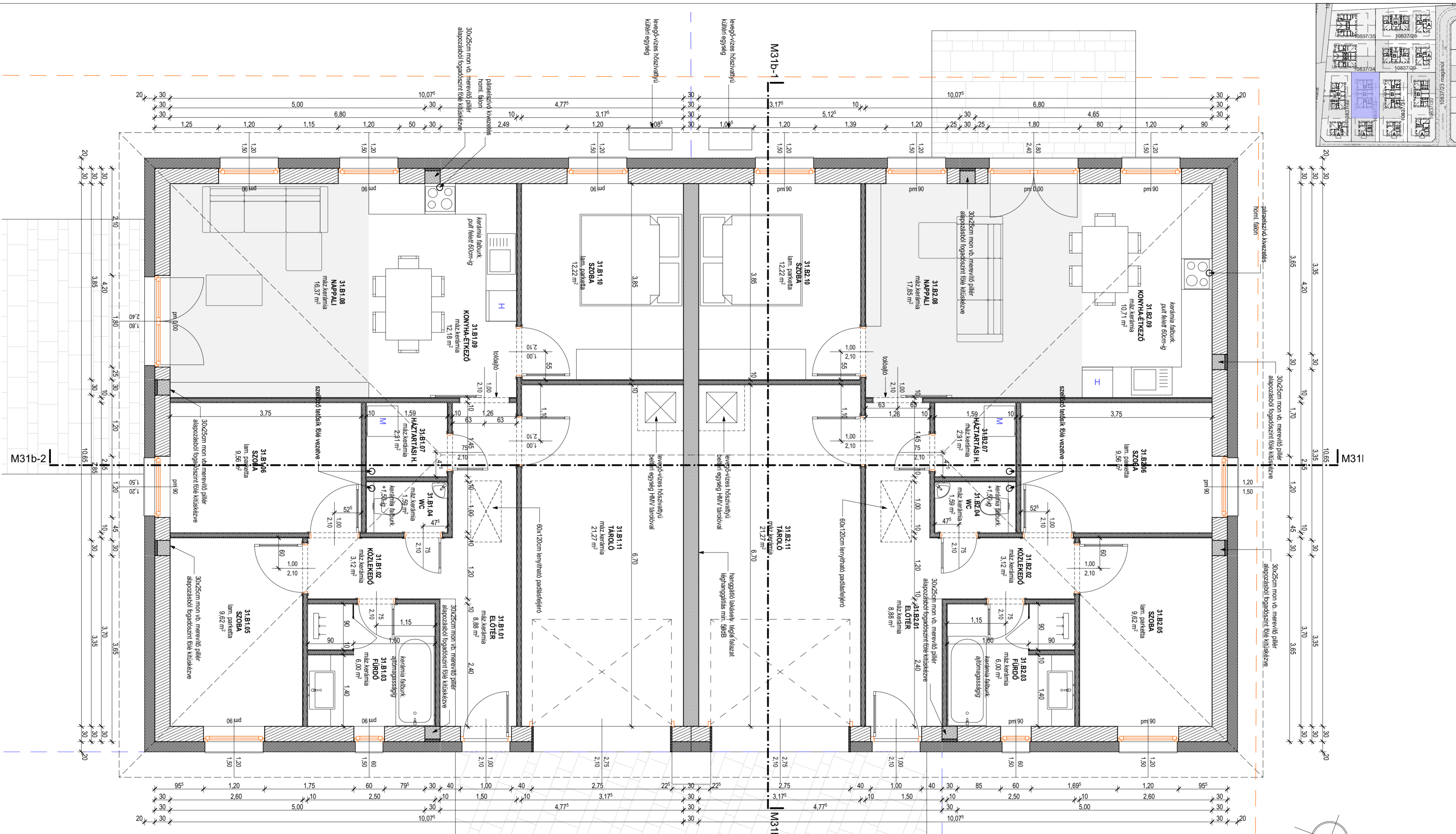
Alaprajz M=1:50
