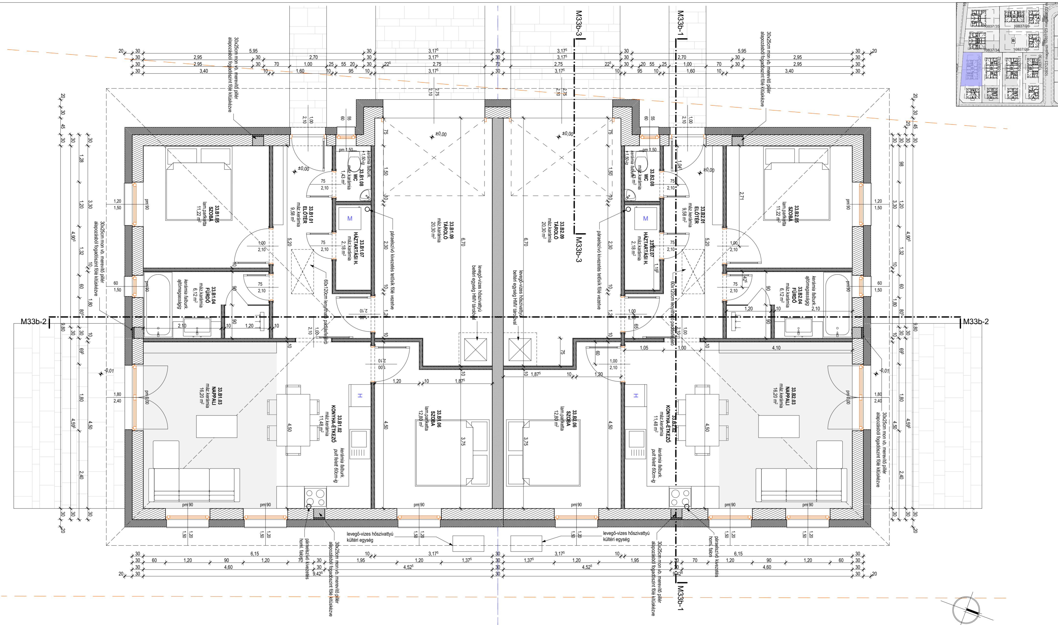
Alaprajz M=1:50
